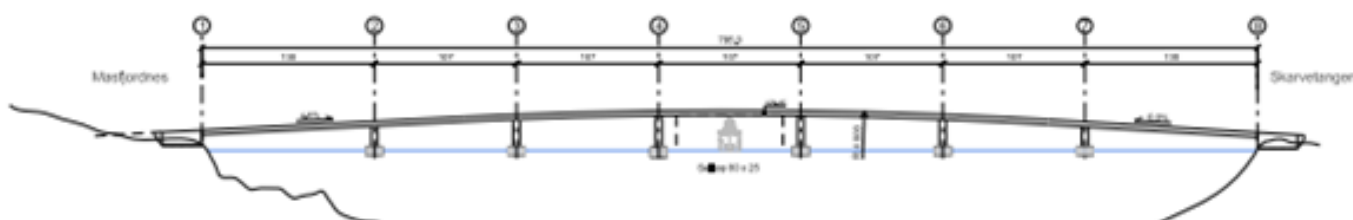
Figur 1: Konseptskisse for flytebru med høgbrekk midtfjords for seilingsløp på 80 x 25 m.
